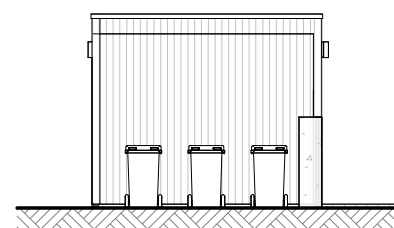
rechtergevel berging type H2/H3 (dubbele)
