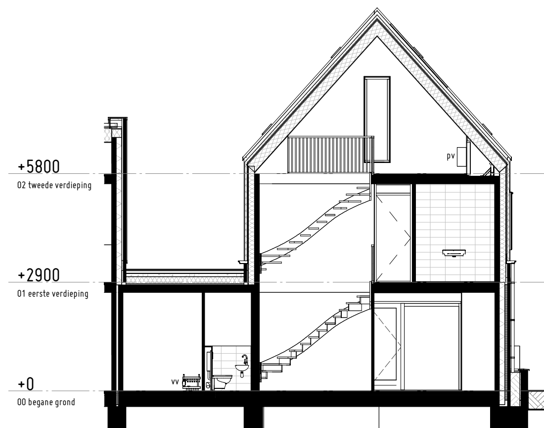
Doorsnede
