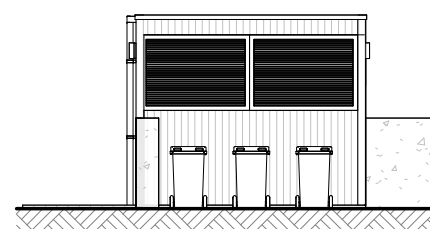
linkergevel berging type H1 (dubbele)
