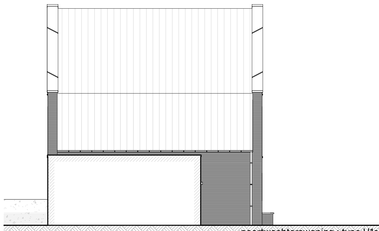
Linkergevel
